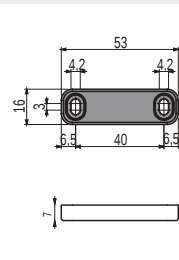
SM L•T actuator
