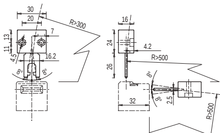
Actuator VF KEYF2
