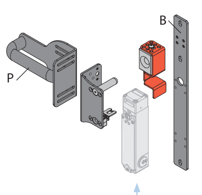
VF AP-P11B-202P
