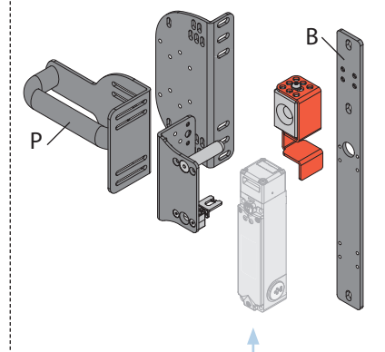
VF AP-P11B-200P
