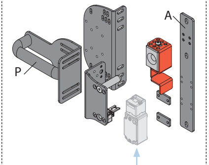
VF AP-P11A-200P
