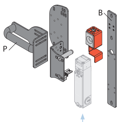
VF AP-P11B-201P
